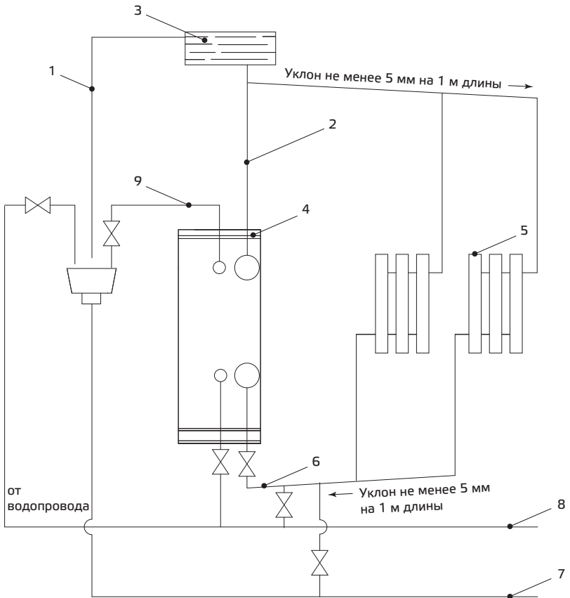
1 — сигнальная труба; 2 — главный стояк; 3 — расширительный бак; 4 — аппарат; 5 — радиатор; 6 — трубопровод обратной воды; 7 — сливная магистраль; 8 — подпиточный водопровод; 9 — трубопровод горячей воды
